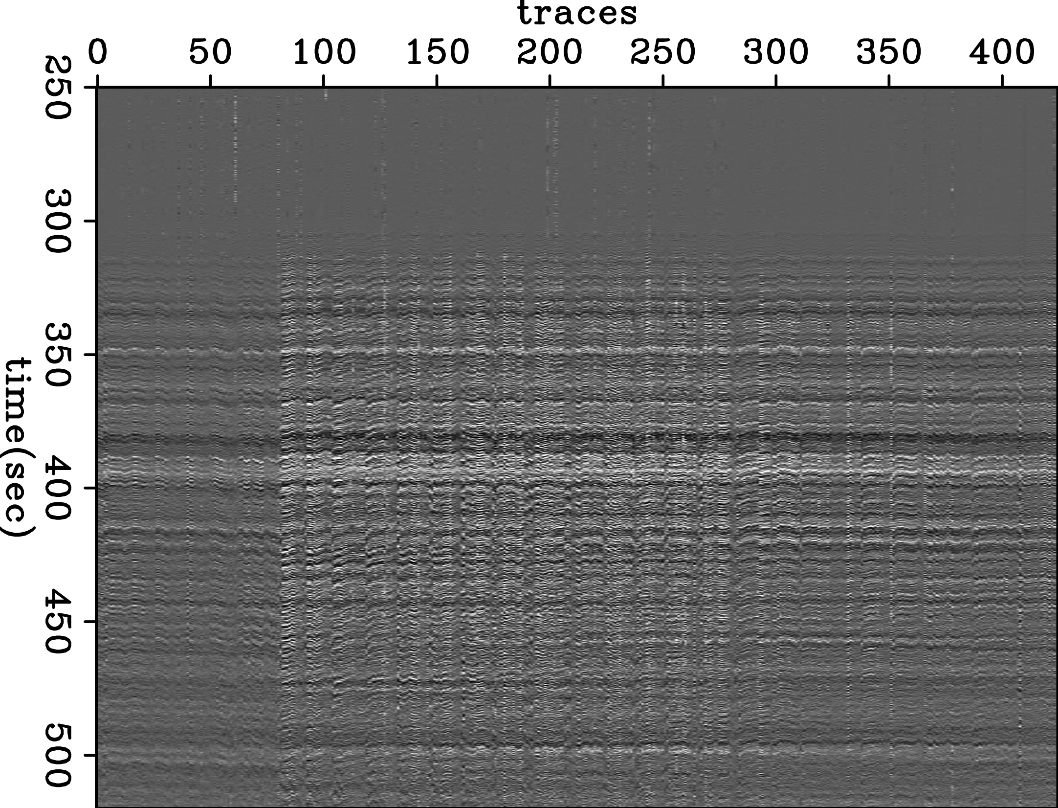
Burg decon(dt=0.125sec len=30)
