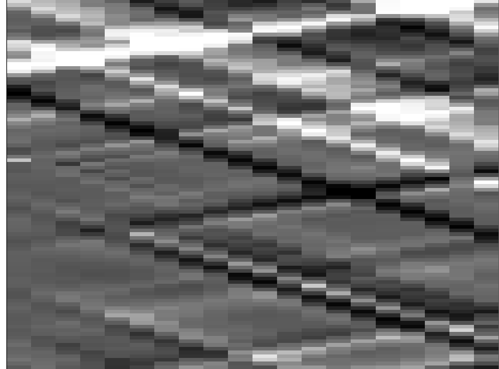
single_scale:_iter=30
