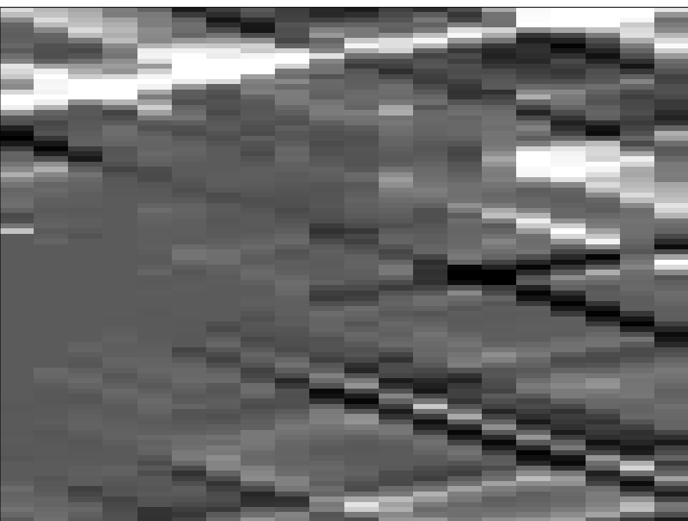
multiscale:___iter=1
