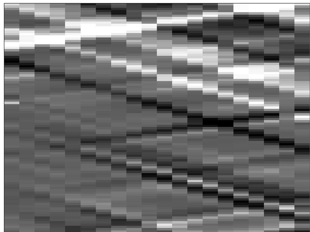
multiscale:___iter=30
