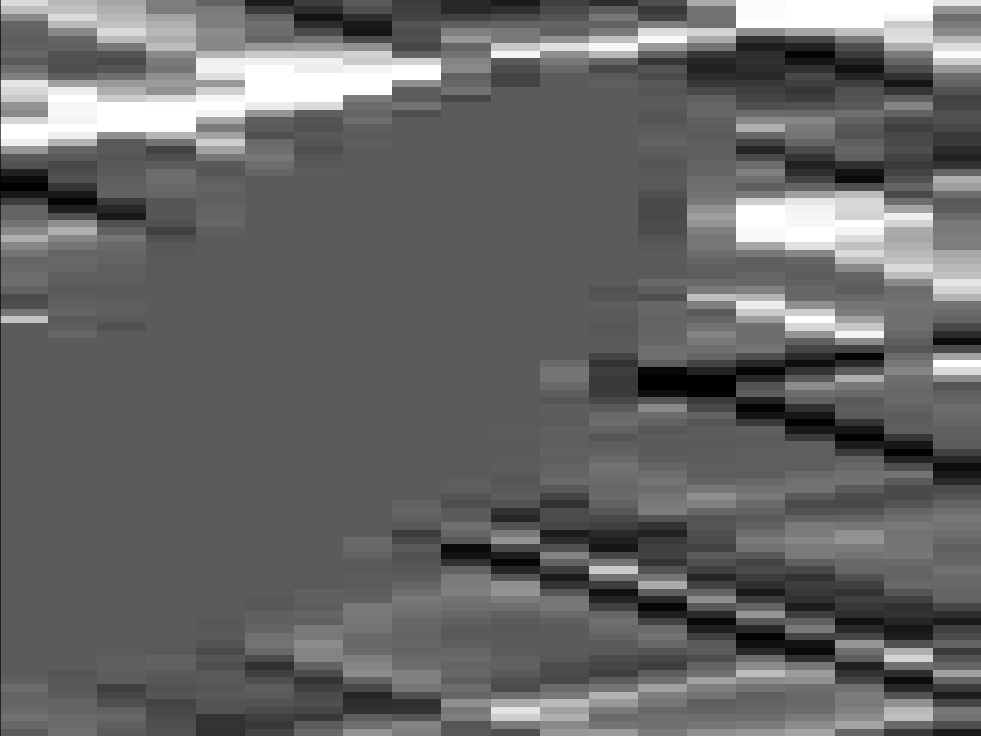
single_scale:_iter=1
