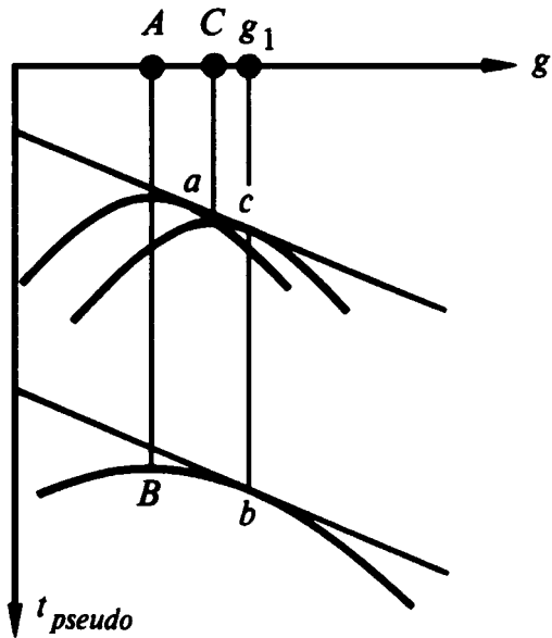
Snell wave
