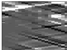
multiscale:___iter=1
