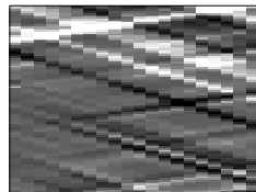
multiscale:___iter=30
