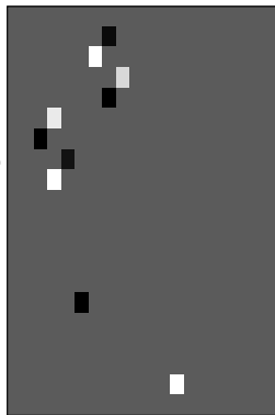
input
