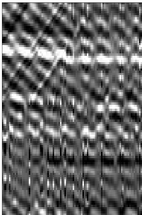
1-axis PEF
