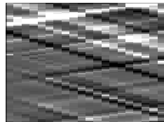
single_scale:_iter=30
