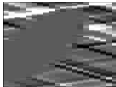
single_scale:_iter=1
