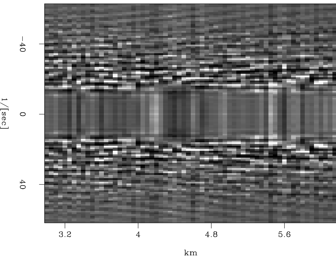
P(\omega,x)
