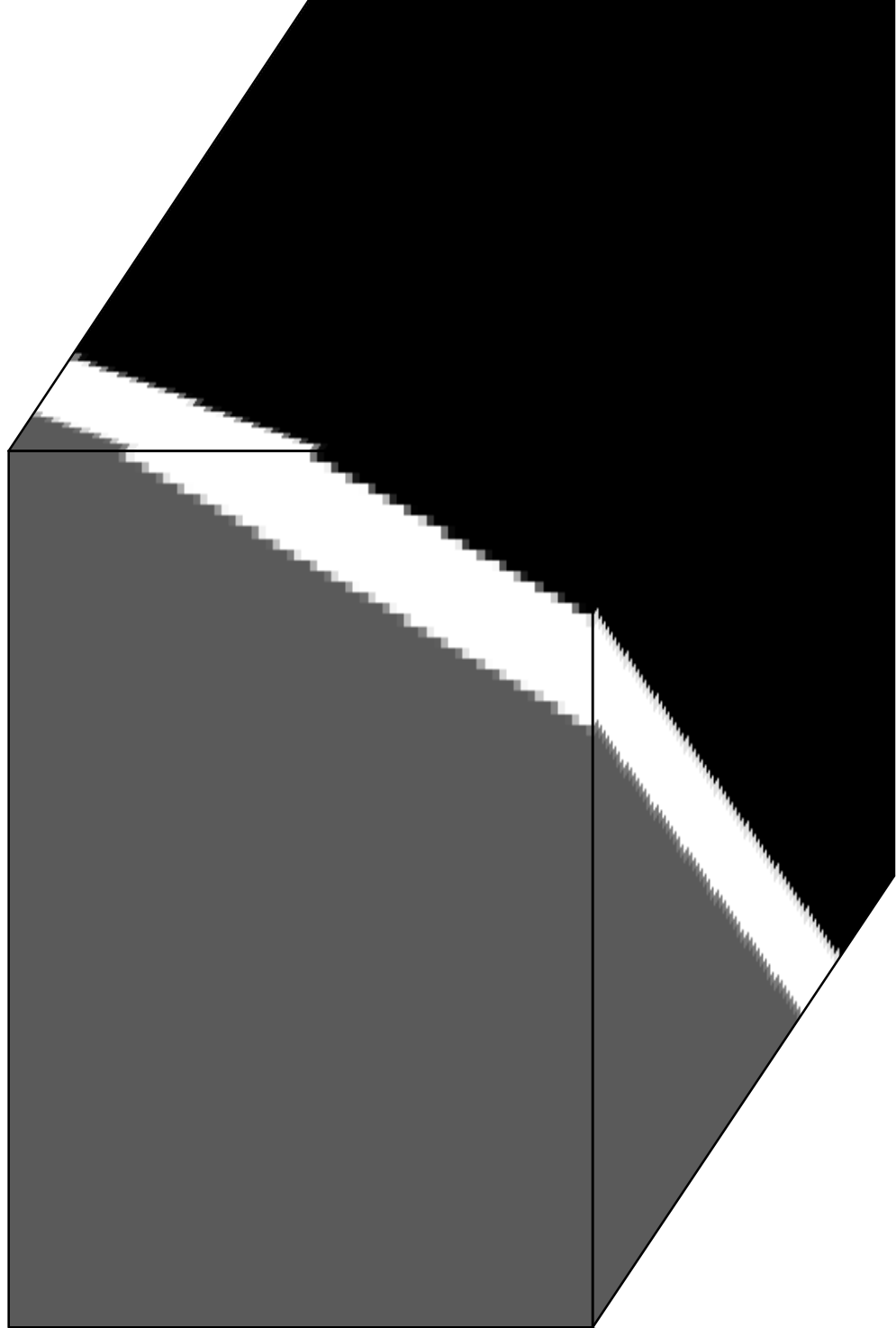
Amplitude edge volume
