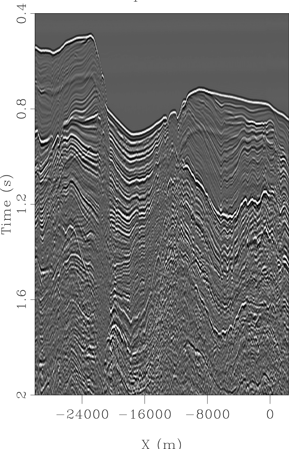
Input data
